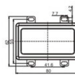
EC控制壳外型尺寸
